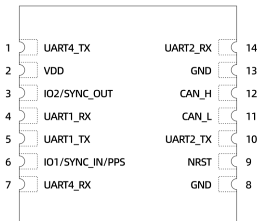
图 4 HI04S2/HI04S3-MI1 引脚定义
