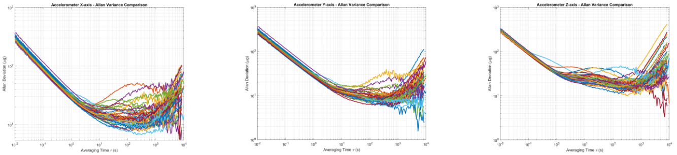
图 14 HI04SX 加速度计艾伦方差
