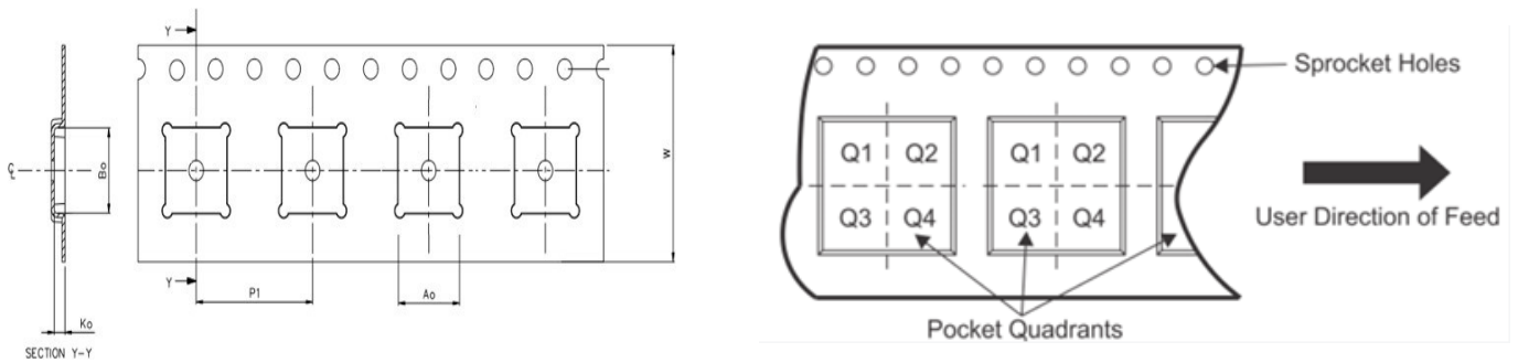
图 20 卷带尺寸与 Pin 1 方向
