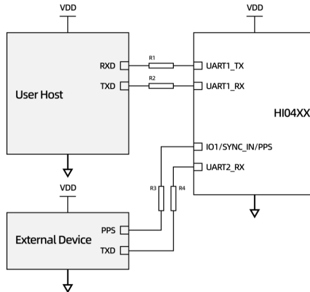
图 10 HI04 与外部设备 PPS + GPRMC 同步
