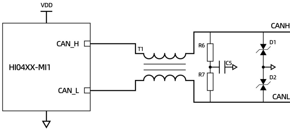
图 8 HI04S2/HI04S3 CAN 通信参考电路
