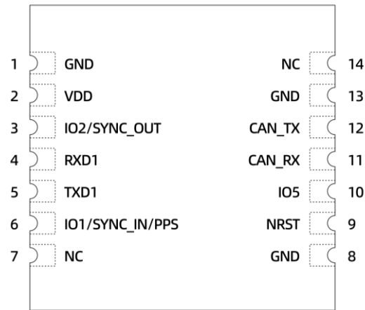
图 3 HI04M0/HI04M3 引脚定义
