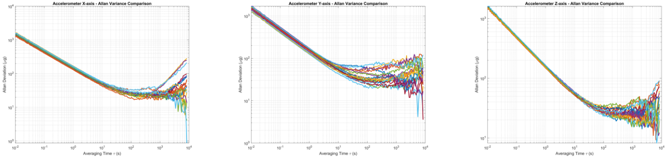
图 13 HI04MX 加速度计艾伦方差
