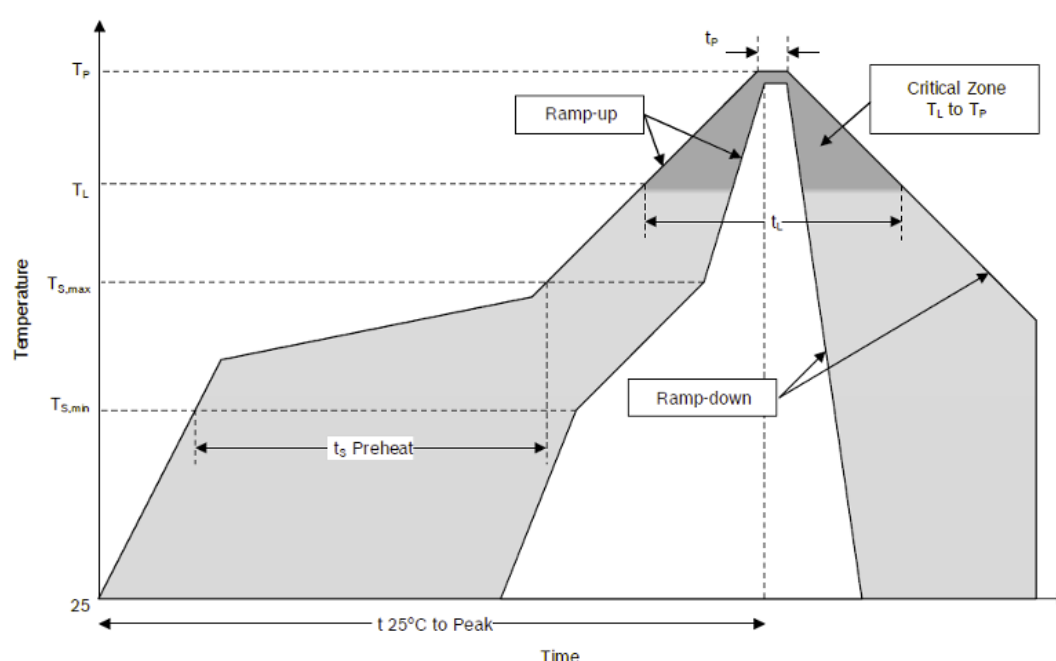
图 19 SMT 温度曲线
