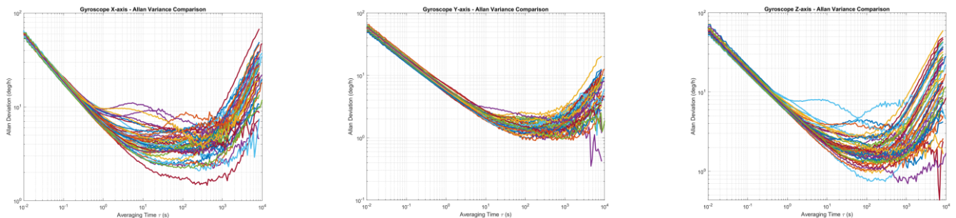
图 12 HI04SX 陀螺仪艾伦方差
