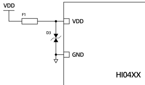
图 5 HI04 电源参考电路
