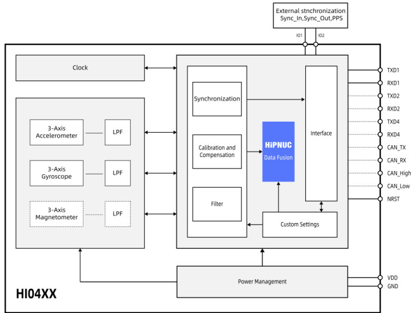
图 1 HI04 系列系统框图
