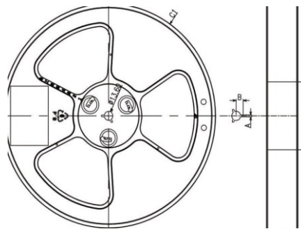
图 21 卷盘尺寸
