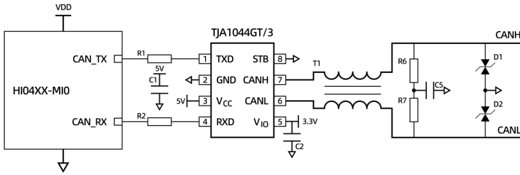
图 7 HI04M0/HI04M3 CAN 通信参考电路
