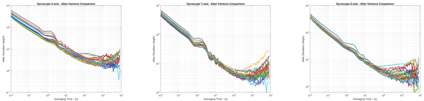
图 11 HI04MX 陀螺仪艾伦方差
