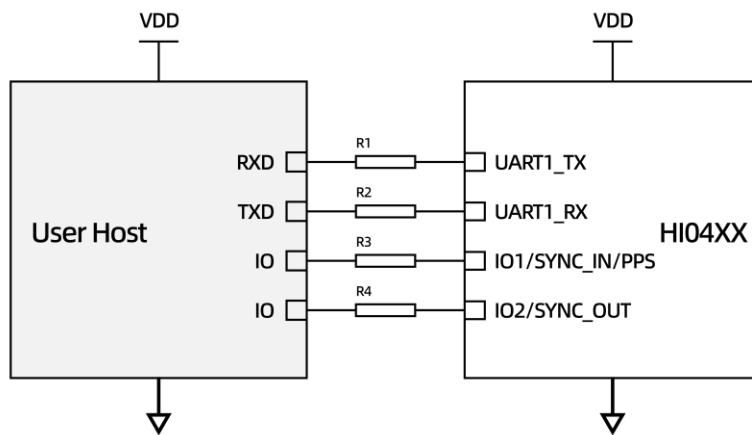
图 9 HI04 与主机触发同步 (串口通信)
