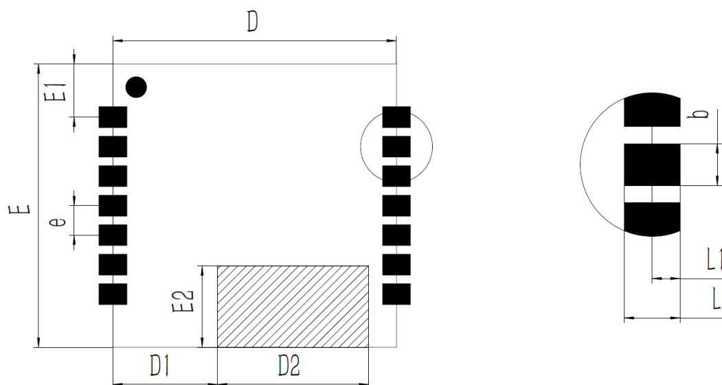
图 16 HI04 推荐的焊盘尺寸
