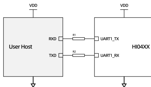
图 6 HI04 串口通信最小系统参考电路
