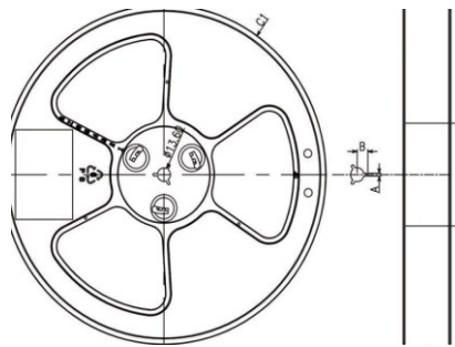
图 21: 卷盘尺寸
