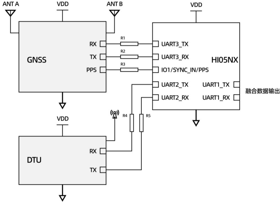
图 11: HI05NX 外接 GNSS
