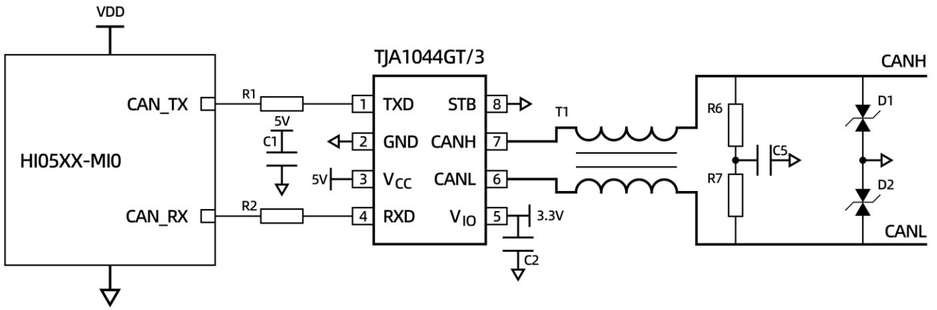
图 7: HI05XX-MI0 CAN 通信电路参考
