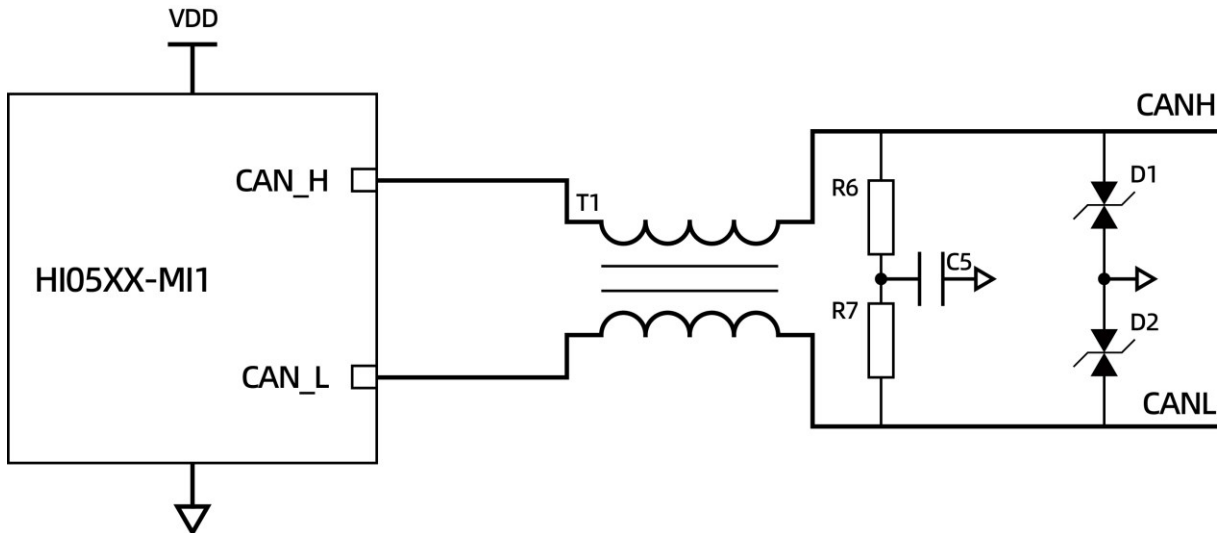
图 8: HI05XX-MI1 CAN 通信电路参考
