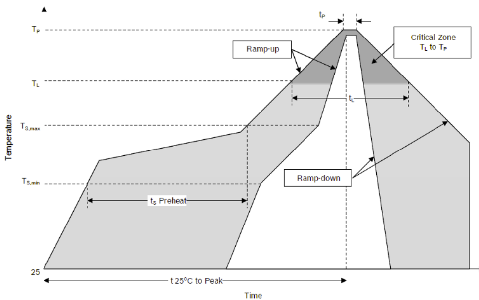
图 19: SMT 温度曲线
