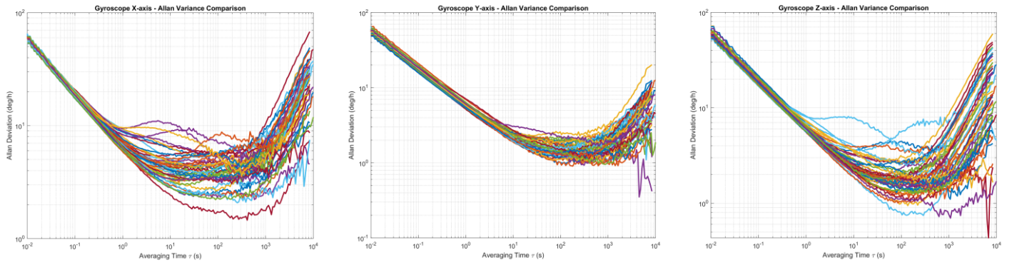
图 12: HI05XX 陀螺仪艾伦方差
