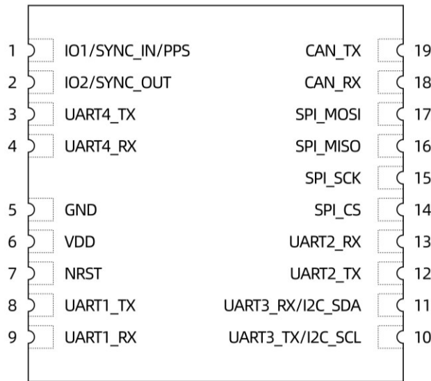
图 3: HI05XX-MIO 引脚定义
