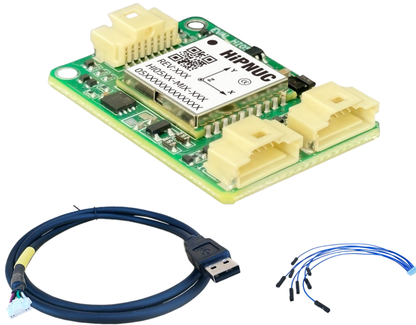
图 18: HI05 系列评估板与线束
