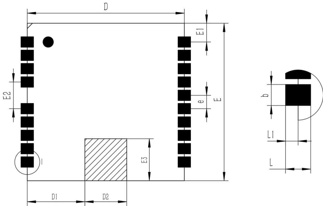
图 15: HI05 推荐的焊盘尺寸
