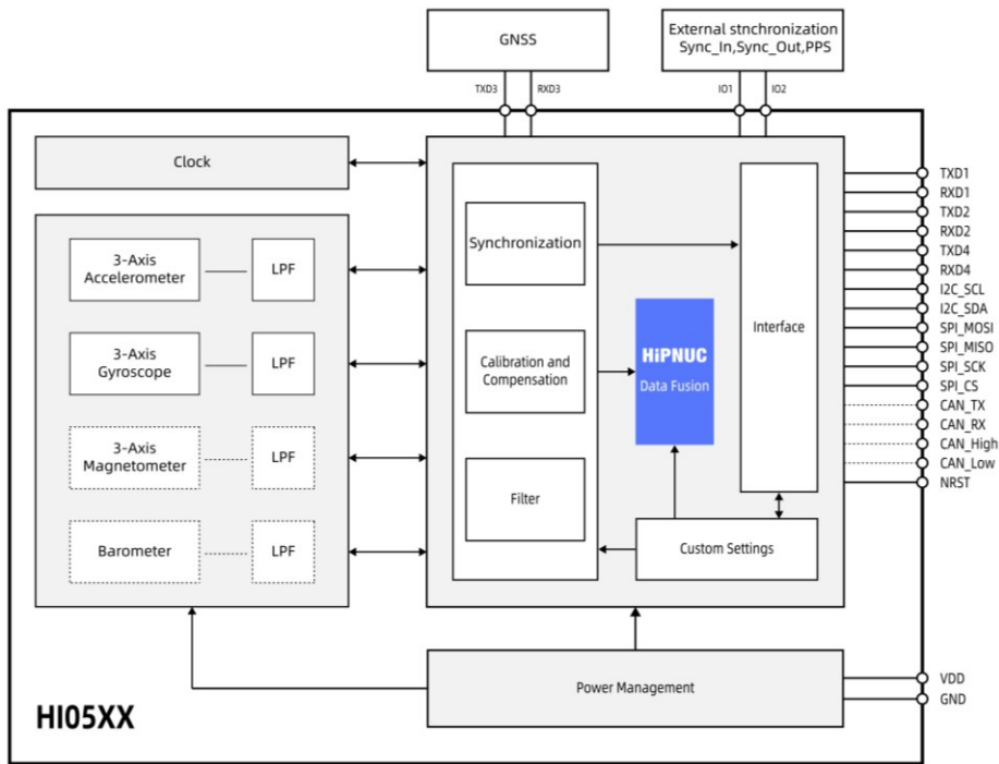
图 1: HI05 系列系统框图
