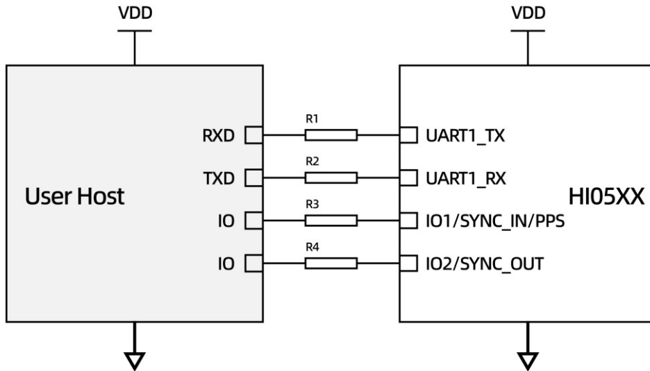
图 9: HI05 与主机触发同步（串口通信）
