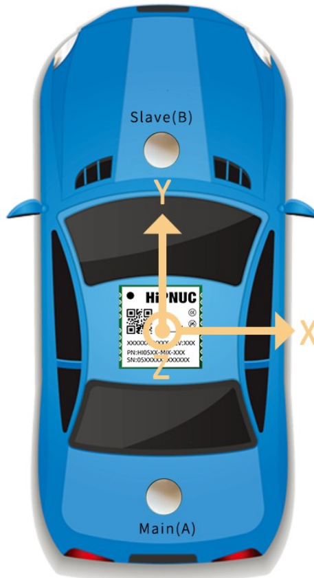
图 17: HI05 外接 GNSS 坐标系定义
