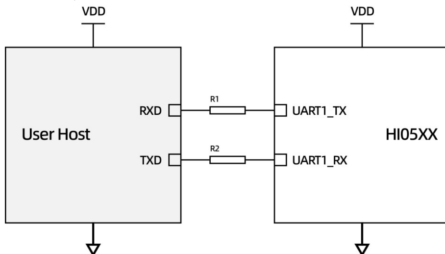
图 6: HI05 串口通信最小系统参考电路
