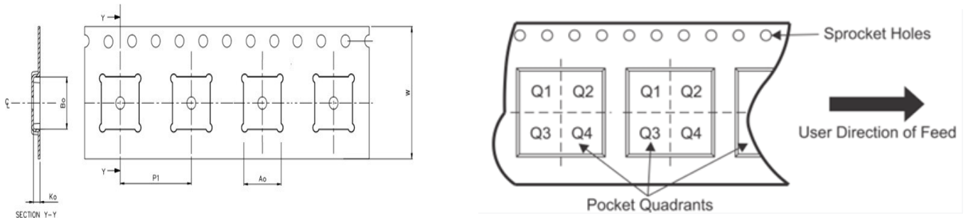
图 20: 卷带尺寸与 1 脚方向
