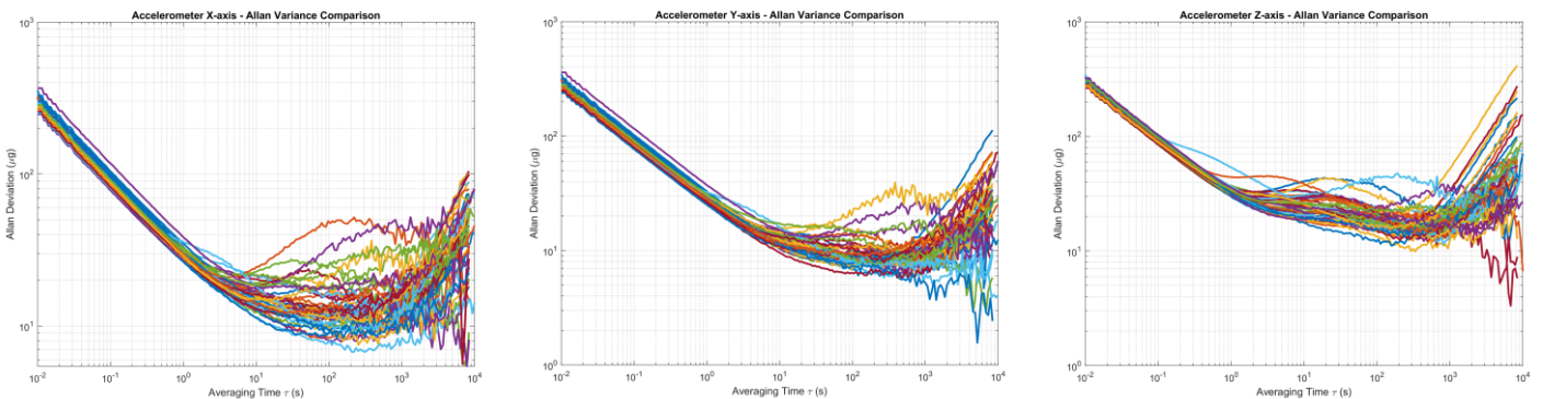
图 13: HI05XX 加速度计艾伦方差
