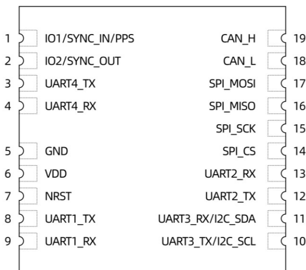
图 4: HI05XX-MI1 引脚定义
