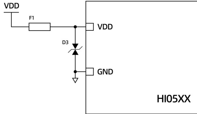
图 5: HI05 电源参考电路
