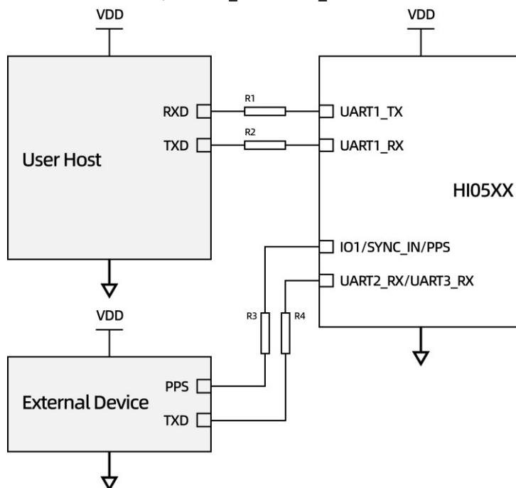
图 10: HI05 与外部设备 PPS+RMC 同步
