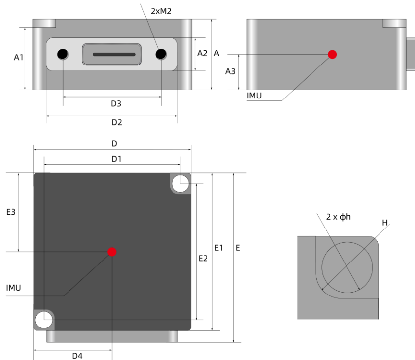
图 9 HI13 机械尺寸与 IMU 位置
