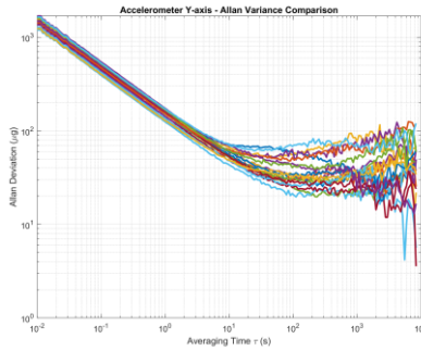
图 6 HI13MX 加速度计艾伦方差
