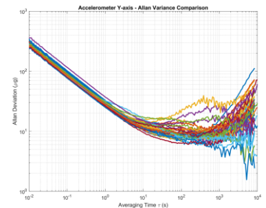
图 8 HI13SX 加速度计艾伦方差
