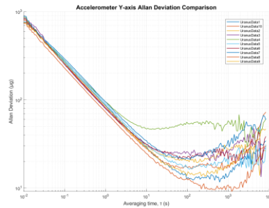
图 7 HI13RX 加速度计艾伦方差
