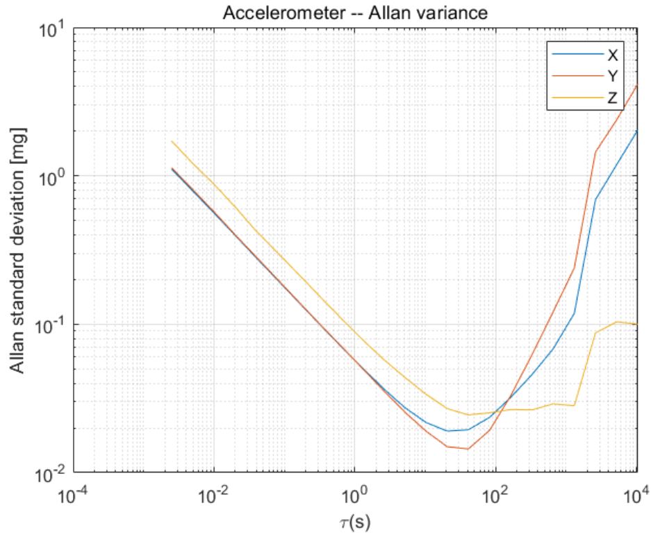
加速度Allan方差曲线
