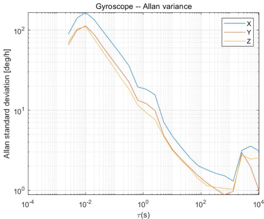
陀螺Allan方差曲线
