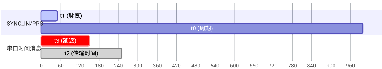
PPS 与串口时间消息时序关系图 (t0-t3)
